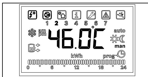
Bild 49 Ausgangsmenü
