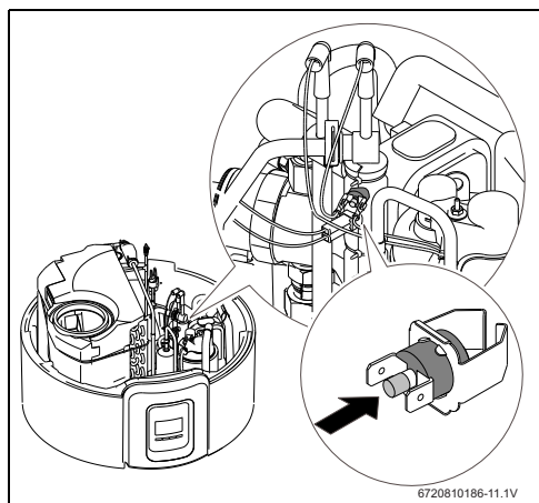
Bild 53 Temperaturbegrenzer
