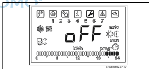
Bild 46 Betriebsart "OFF"
