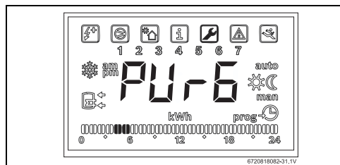
Bild 38 Funktion "Purg"
