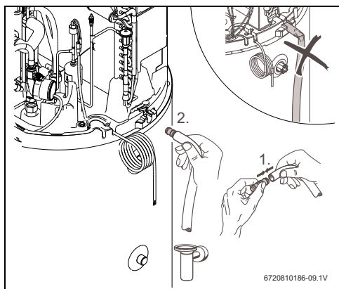
Bild 12 Kondensatabfang
