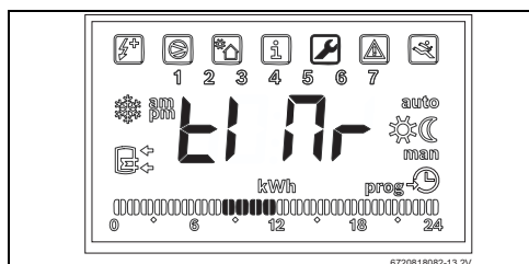
Bild 24 Untermenü "Timr"
