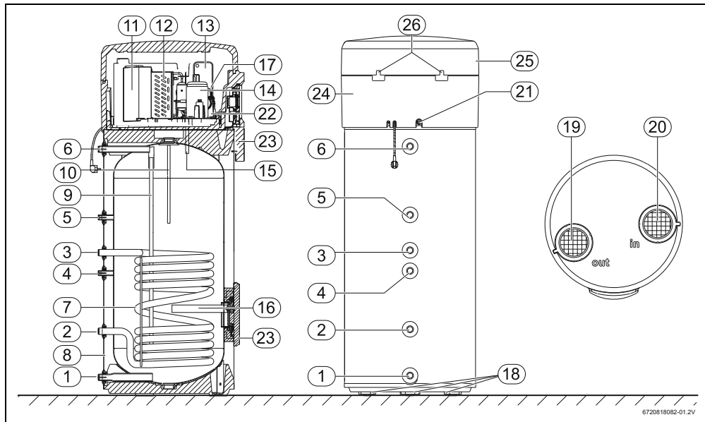
Bild 3 Wärmepumpe
