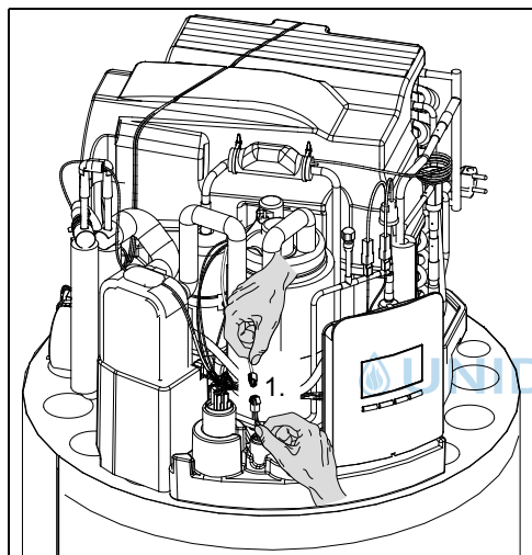
Bild 50 Gebläse-Anschlusskabel
