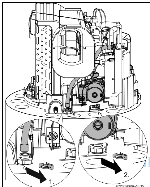
Bild 53 Haltefeder abnehmen
