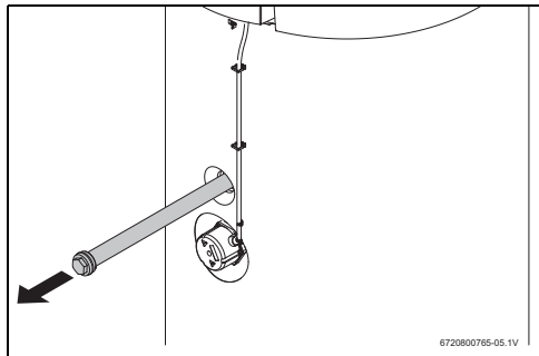
Bild 54 Kontrolle des Zustands der Magnesium-Anode
