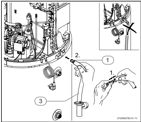
Bild 12 Kondensatauffang
