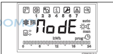
Bild 22 Funktion „Mode“
