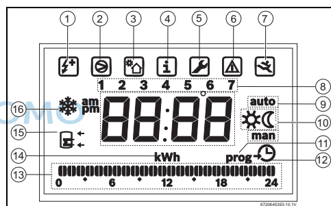
Bild 15 Anzeige
