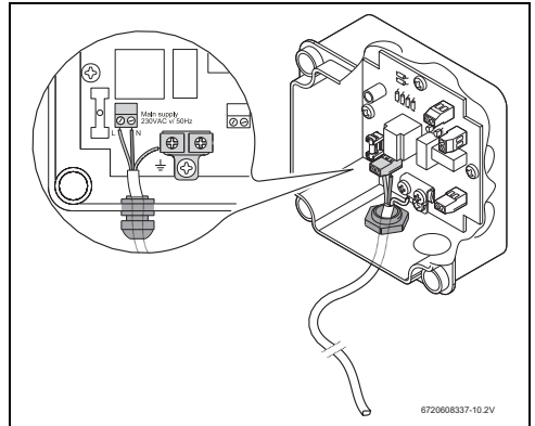
Bild 16 Netzananschluss 230 VAC
