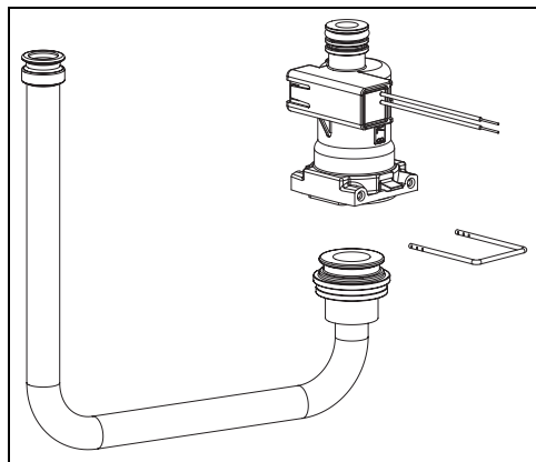
Bild 8 Zusammenbau
