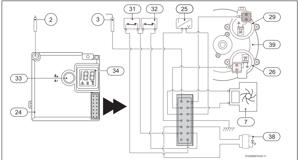
Bild 5 Elektrische Verdrahtung
