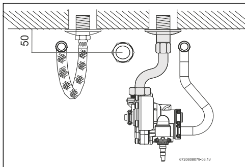
Bild 8 Unterputz-Installation
