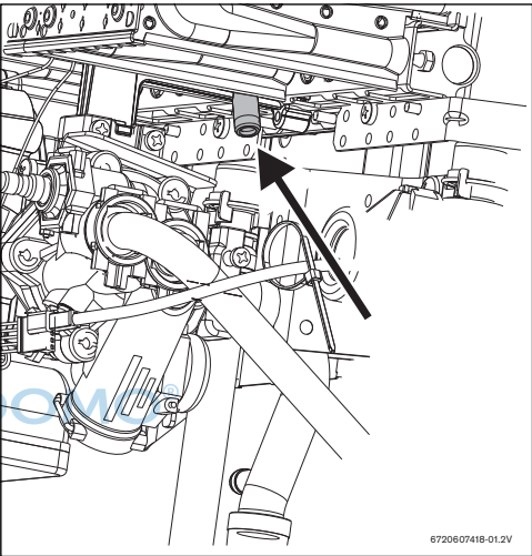
Bild 18 Messpunkt Düsendruck
