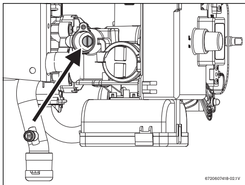
Bild 19 Einstellschraube max. Gasmenge
