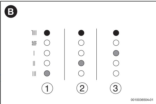
4 de: Störung (rote und gelbe LED) / en: fault (red and yellow LED) [1] de: Rotor blockiert / en: Rotor is blocked [2] de: Netzspannung zu niedrig / en: supply voltage too low [3] de: Störung der Electronik / en: electrical error
