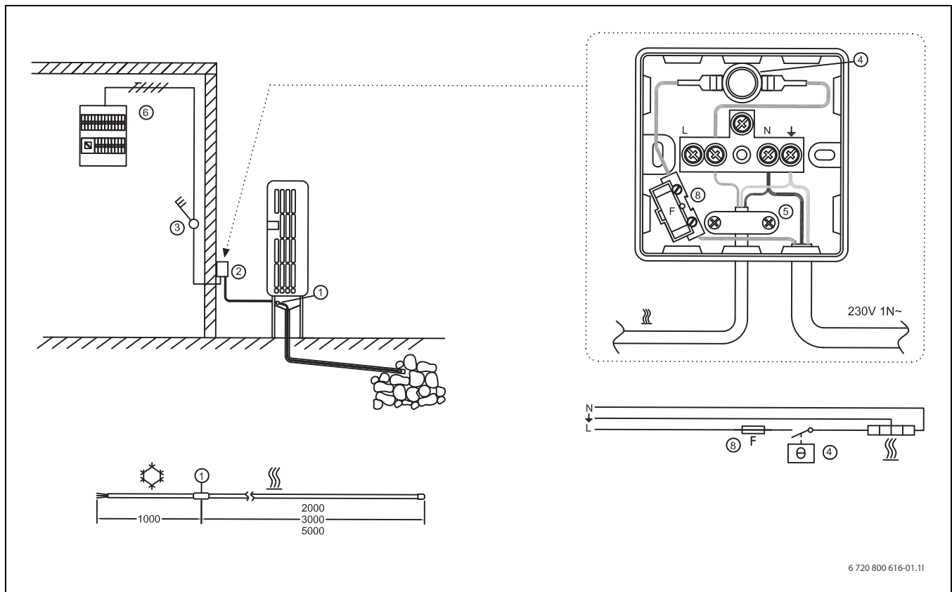
Pav. 37 Šilumos siurblys su vandens linija tarp vidinės ir išorinės dalies prijungimo nurodymai
