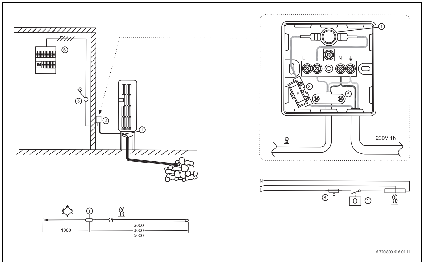
Rys. 46 Wskazówki dot. podłączenia dla pompy ciepła z przewodem wodnym między częścią wewnętrzną i zewnętrzną
