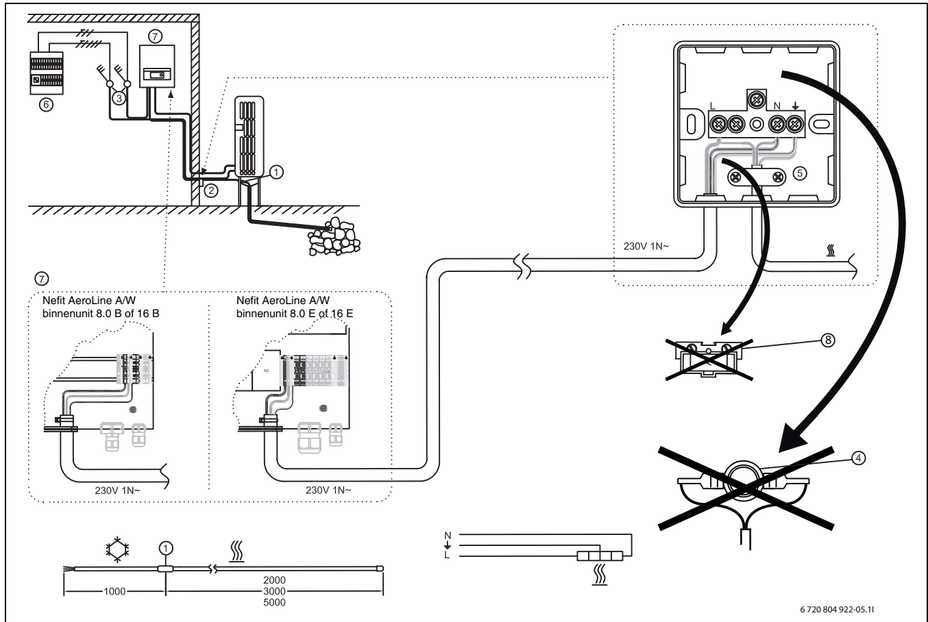
Afb. 11 Aansluitschema verwarmingskabel
