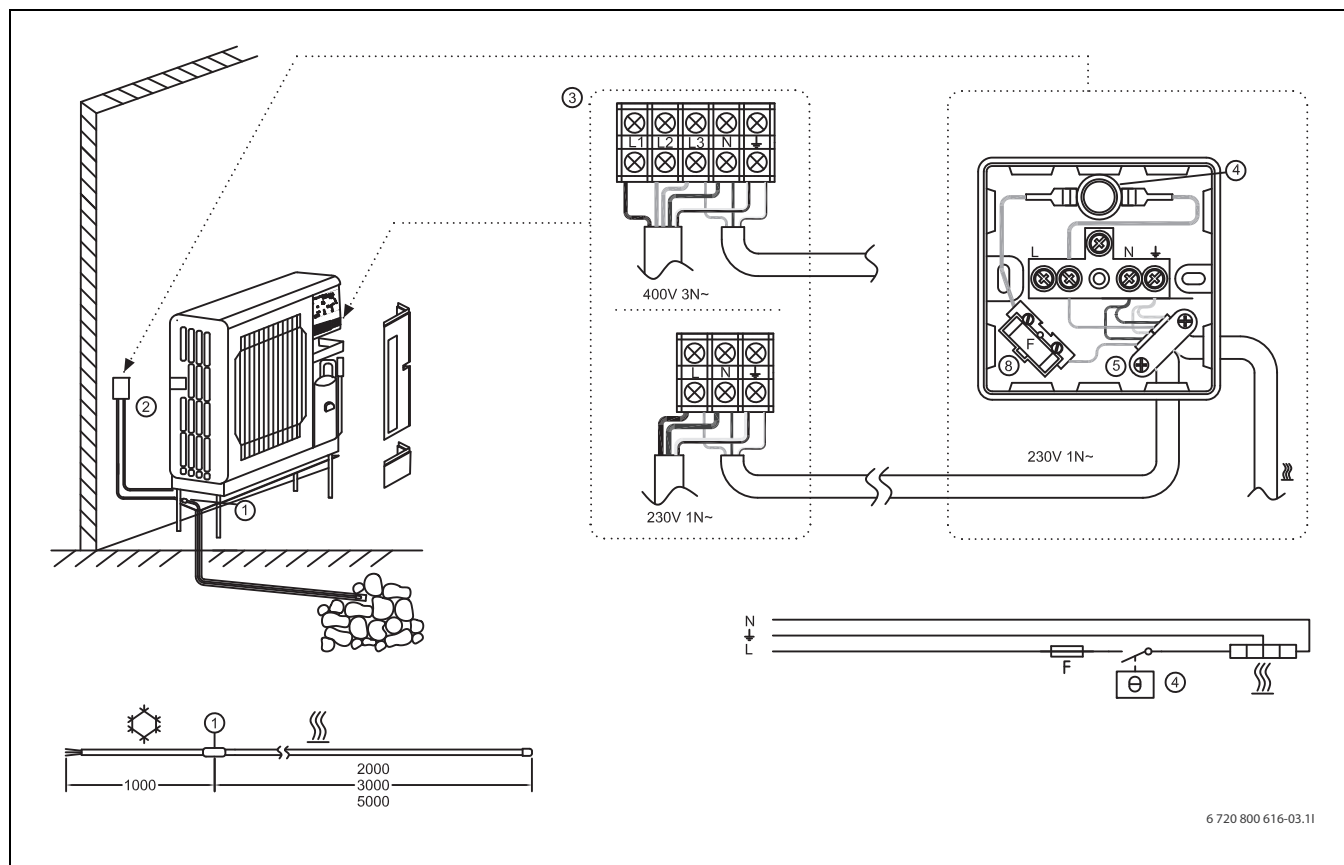
Joon. 18 Sise- ja välisosa vahelise vektoruga või jahutusaine läbivoolutoruga soojuspumba ühendamise juhised.
