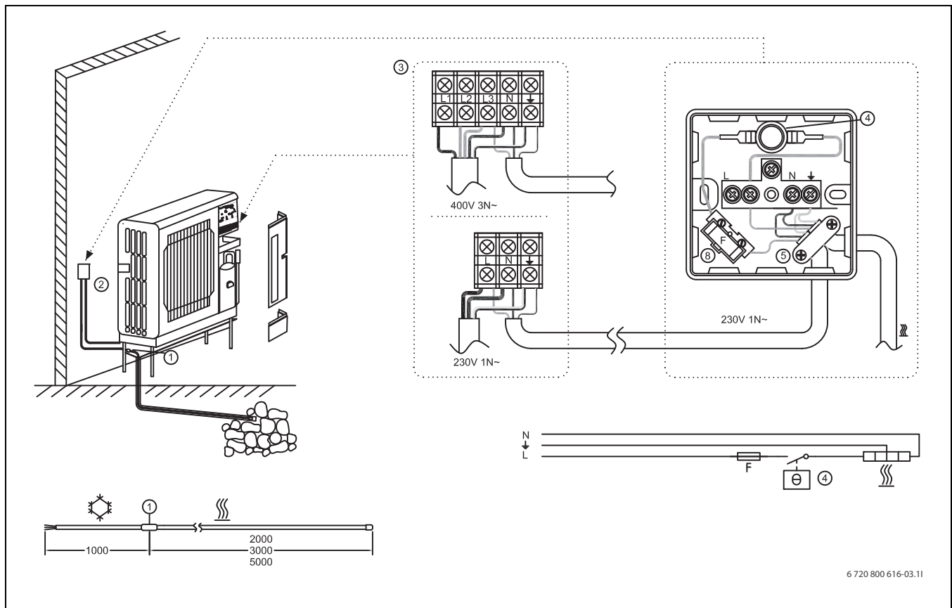
Afb. 12 Aansluitschema verwarmingskabel
