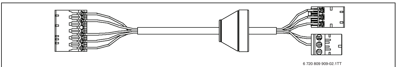
Bild 3 Netzleitung bis 04/2014 ohne Ferritkern
