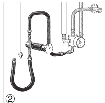
Anschlussset mit UP-Rohrunterbrecher DN 20 (Bauart A2, DIN 1988-4) oder (DIN EN 1717) Modell 6161.86
