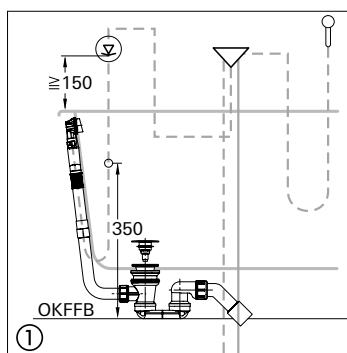
Einbauschema
