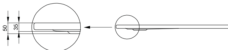
Duschanne mit Schenkel > 1000 mm
