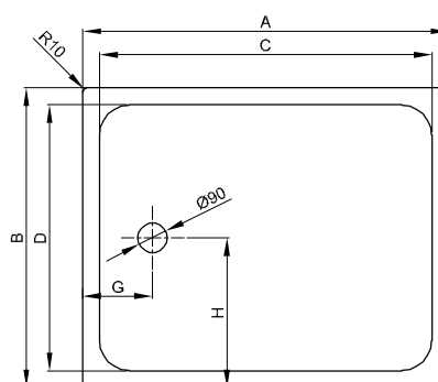
Duschanne mit Schenkel \geq 1000 mm
