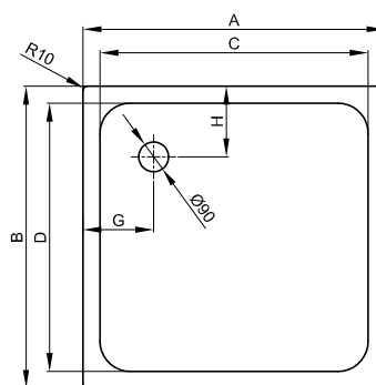
Duschanne mit Schenkel < 1000 mm
