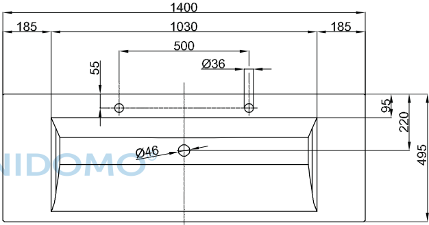
Abb.: BetteAqua 1400 x 495 mm mit 2 Hahnlöchern
