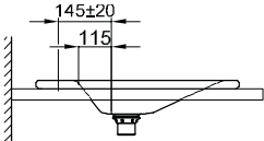
Armaturenempfehlung: Ausladung Armatur: ca. 145 mm ab Mitte Hahnloch
