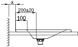
Armaturenempfehlung: Ausladung Armatur: Wandabstand x mm + ca. 200 mm ab Außenkante
