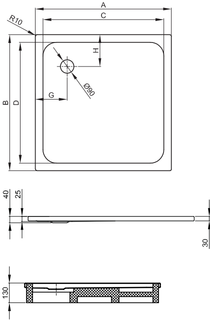
Darstellung mit Wannenträger
