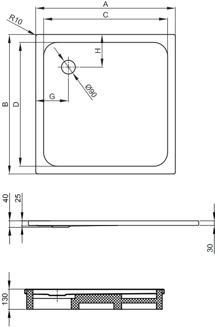
Darstellung mit Wannenträger
