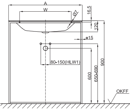
Montage- und Anschlussmaße:
