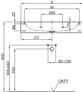
Montage- und Anschlussmaße:
