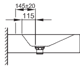
Armaturenempfehlung: Ausladung Armatur: ca. 145 mm ab Mitte Hahnloch
