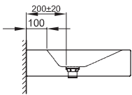
Armaturenempfehlung: Ausladung Armatur: ca. 200 mm ab Wand
