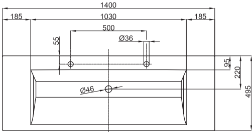
Abb.: BetteAqua 1400 x 495 mm mit 2 Hahnlöchern
