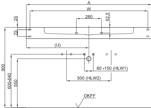
Montage- und Anschlussmaße:
