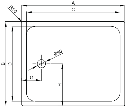
Duschwanne mit Schenkel ≥ 1000 mm
