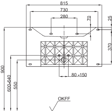
Montage- und Anschlussmaße:
