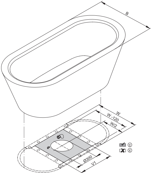
Anschlussmaße für Ab- und Überlaufgarnitur
