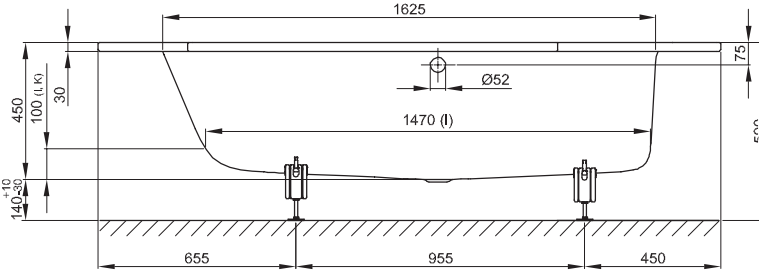
N° 2: Fußende links, Überlauf vorne, Bestell-Nr. 6841
