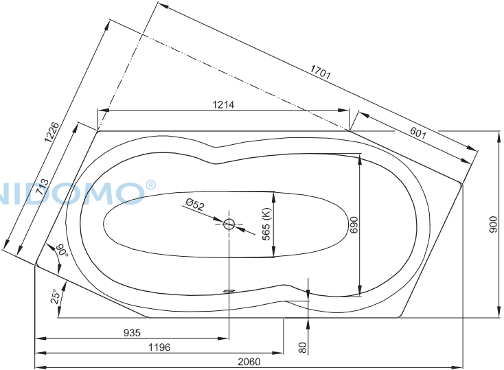
N° 2: Fußende links, Überlauf vorne, Bestell-Nr. 6841
