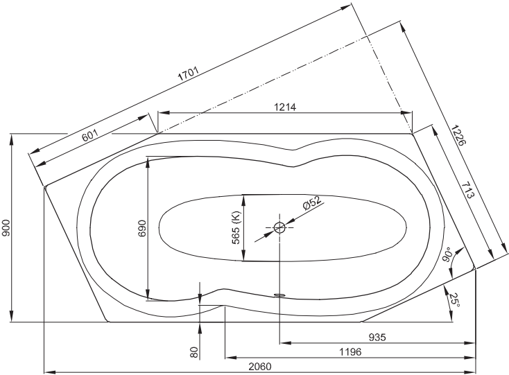
N° 1: Fußende rechts, Überlauf vorne, Bestell-Nr. 6840
