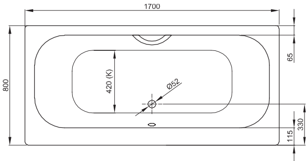
1700 x 800 mm, asymmetrischer Wannenrand, Bestell-Nr. 3100
