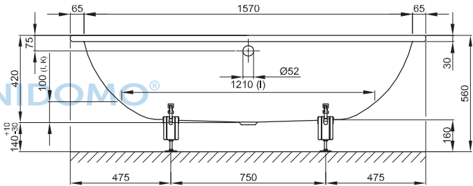
1700 x 800 mm, asymmetrischer Wannenrand, Bestell-Nr. 3100
