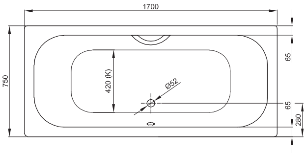
1700 x 750 mm, Bestell-Nr. 3020
