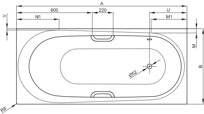
N° 2: Fußende rechts, Überlauf hinten
