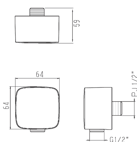
完成図
