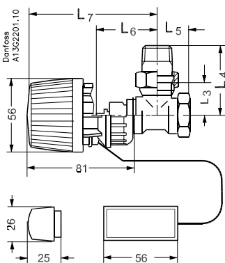
Element mit Fernfühler. Gehäuse in Eckausführung.
