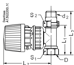
Element mit eingebautem Fühler. Gehäuse in Ausführung Durchgang.
