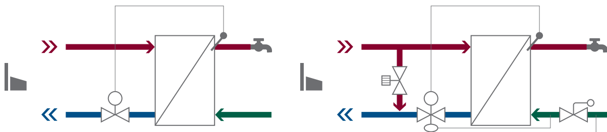
Beispiel für selbsttätige Regelungen
