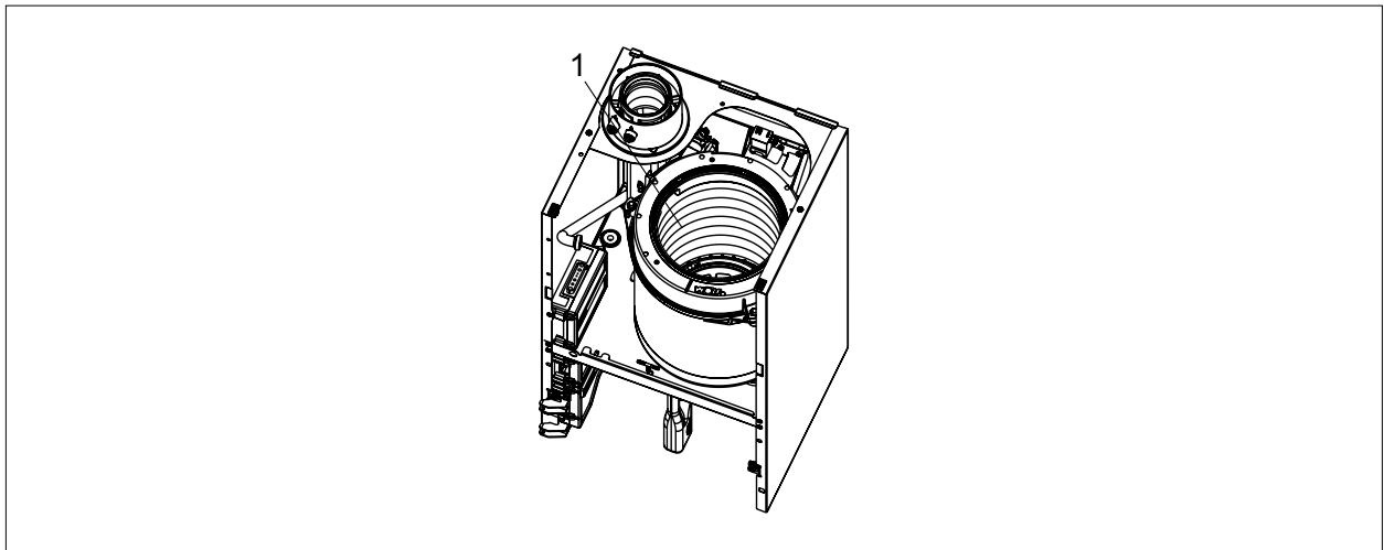
Abb. 6.9 Wärmetauscher reinigen
