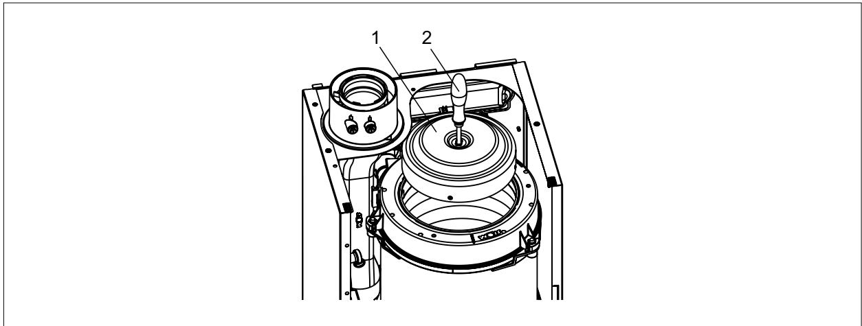
Abb. 6.8 Brennkammertopf-Unterteil ausbauen
