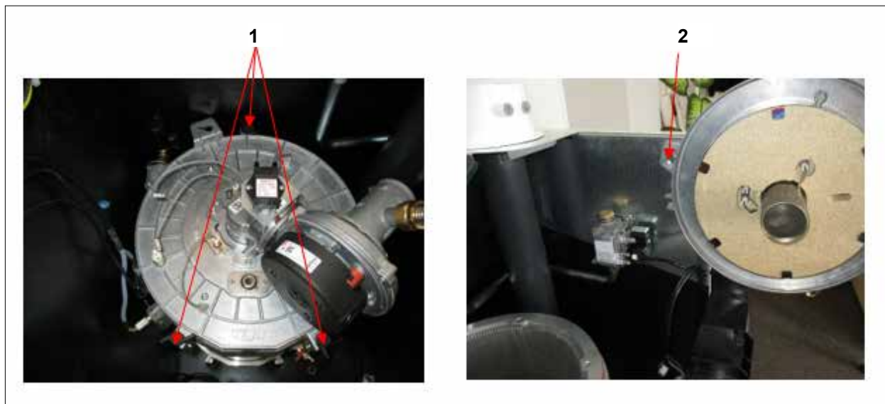
Abb. 5.11 Brennerdeckel Wartungsposition
