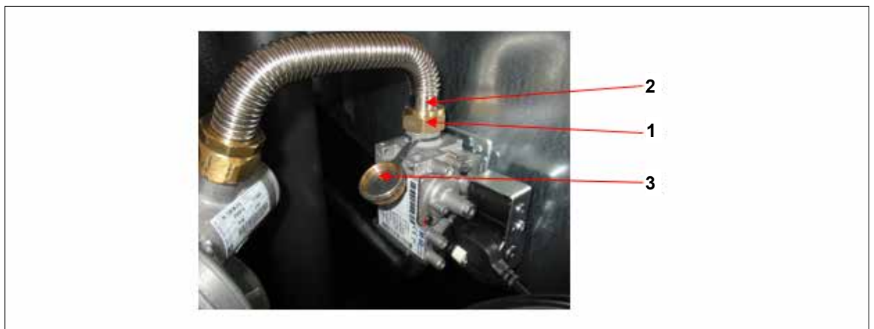
Abb. 5.24 Gaswellrohr anschliessen
