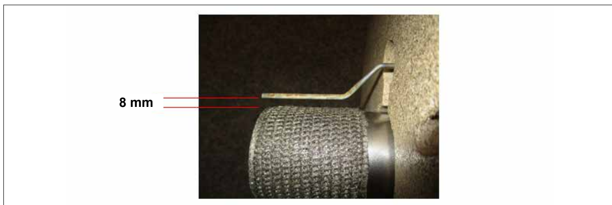
Abb. 5.12 Abstand Ionisationselektrode
