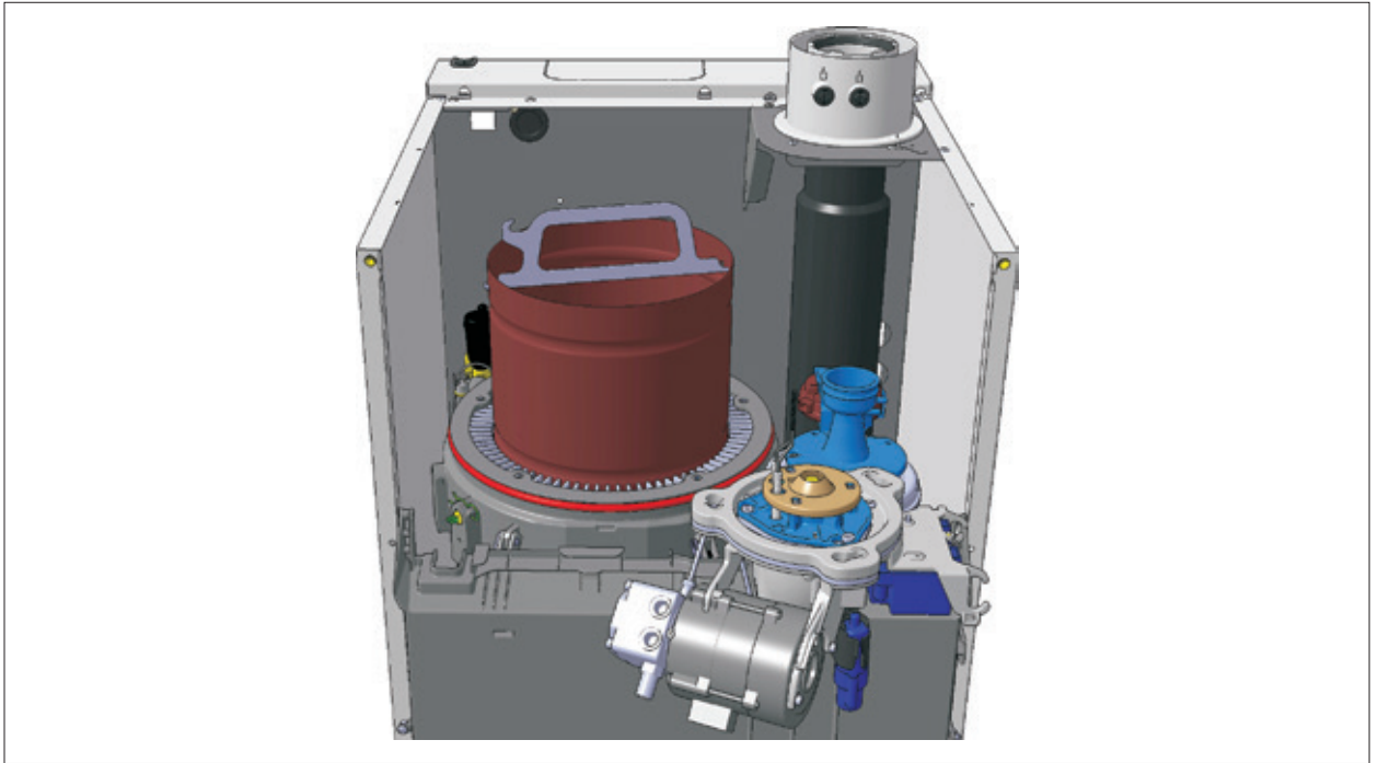
Abb. 4.14 Brennkammer herausziehen
