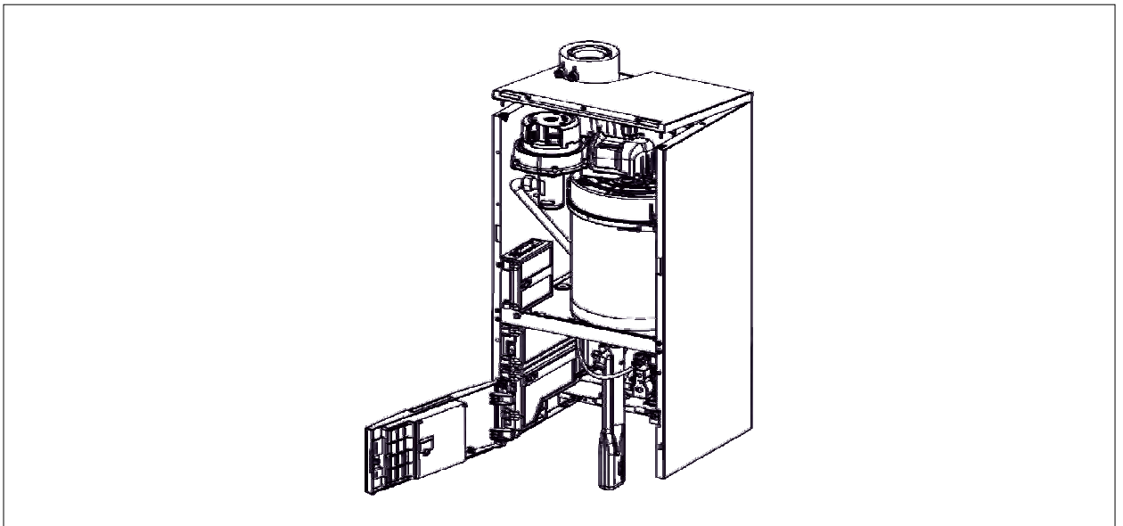
Abb. 5.5 Gerätedeckel abnehmen
