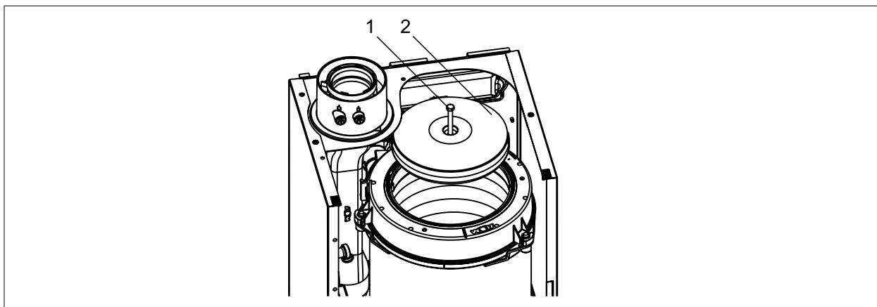
Abb. 6.6 Brennkammertopfoberteil
