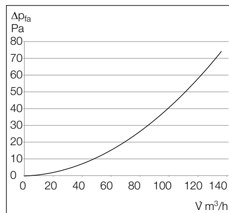
Druckverlust-Volumenstrom Type VFE 70 Type VFE 90
