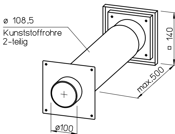
TMK 100 Mauereinbau / Wall Installation / Installation murele
