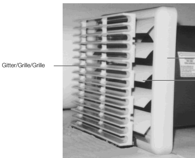
TMK 100 Mauereinbau / Wall Installation / Installation murele
