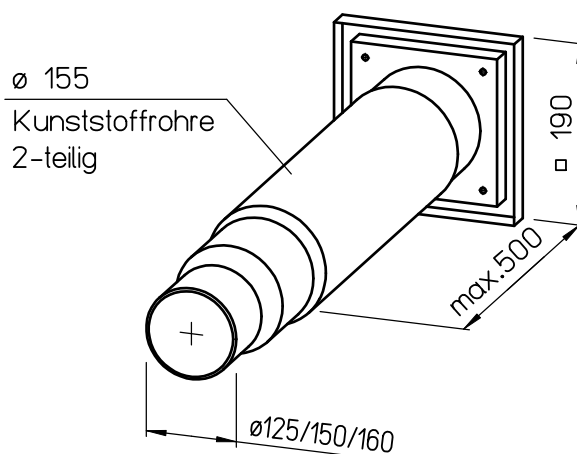
TMK 125 / 150 / 160 Mauereinbau / Wall Installation / Installation murele
