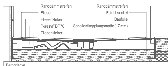
Schematische Schnittzeichnung
