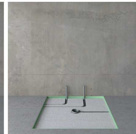
2. Einbau des Unterbauelements und des Bodenablaufs. Für die Rohrleitungen werden entsprechende Aussparungen geschnitten.
