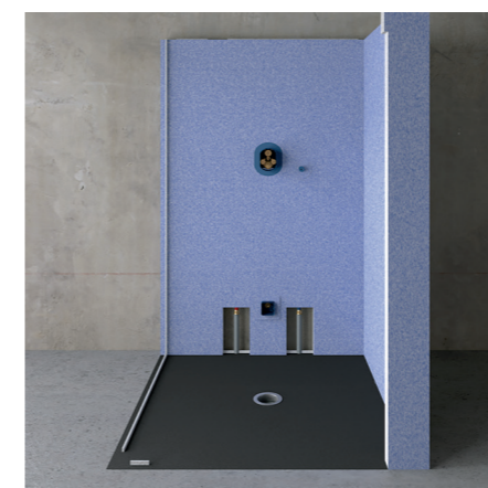
4. Montage der Wandelemente mittels Verbindungsfedern und Verbinder unter Verwendung von Montagekleber. Anschließen von Wasser und Abwasser, Druckprobe!
