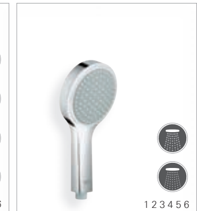
27 660 000 Handbrause 115 2 Strahlarten: Rain, GROHE Rain O 2 27 661 000 mit Durchflusskonstanthalter 9,5 l/min
