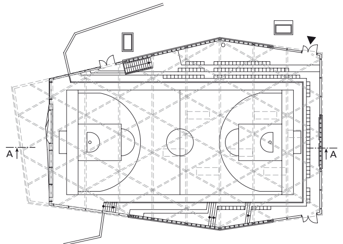
Grundriss Erdgeschoss, M 1:500
