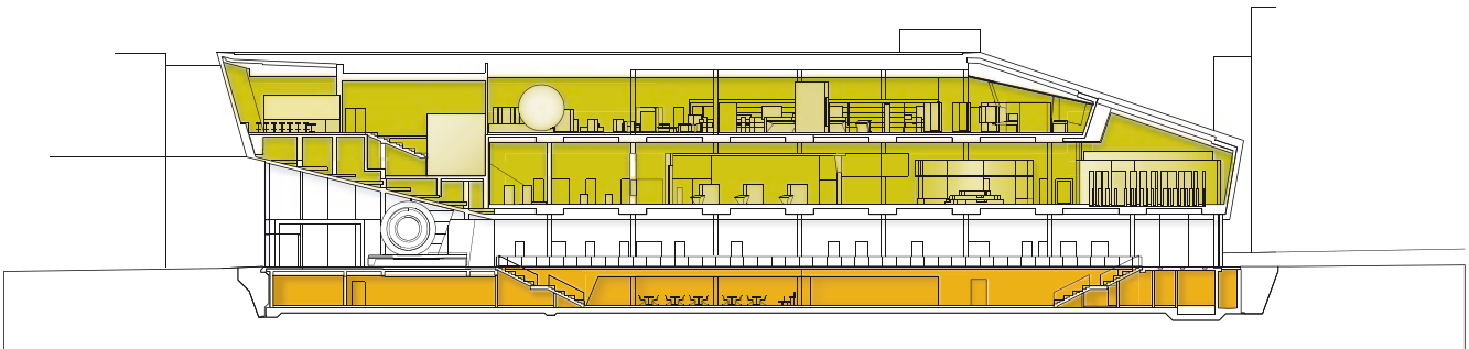
Längsschnitt, M 1:750
