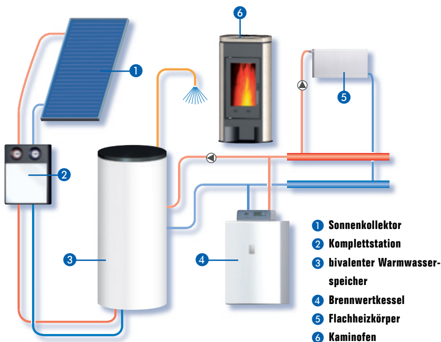
Beispiel für die Erweiterung einer Heizungsanlage durch den Einsatz regenerativer Energien
