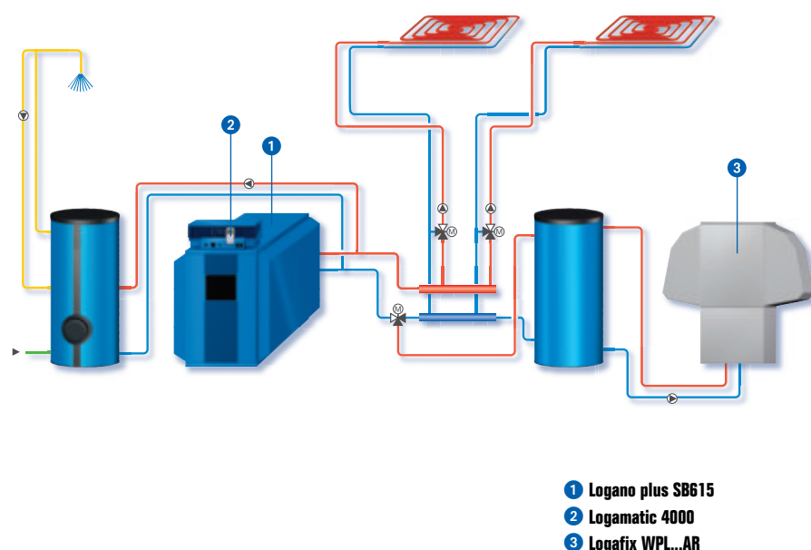
Hydraulisches Systembeispiel
