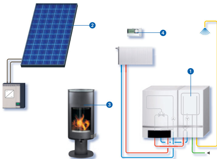
Hydraulisches Systembeispiel
