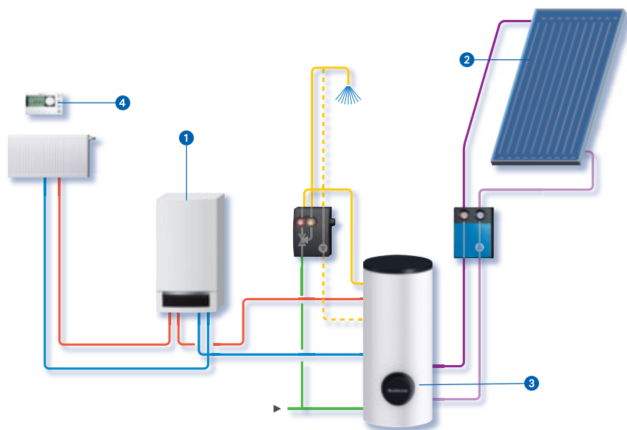
Hydraulisches Systembeispiel
