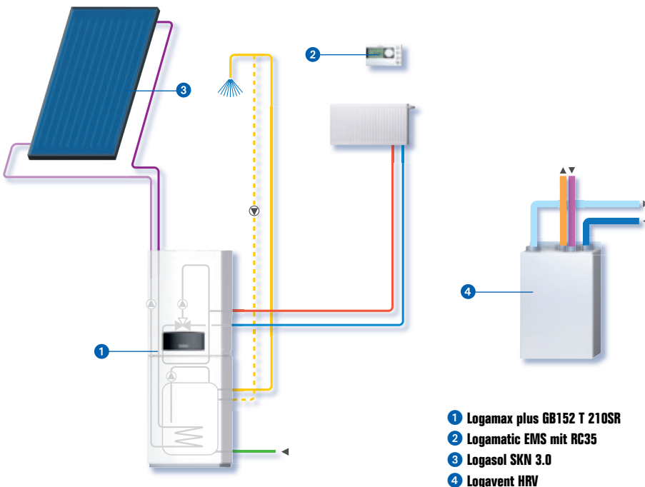
Hydraulisches Systembeispiel
