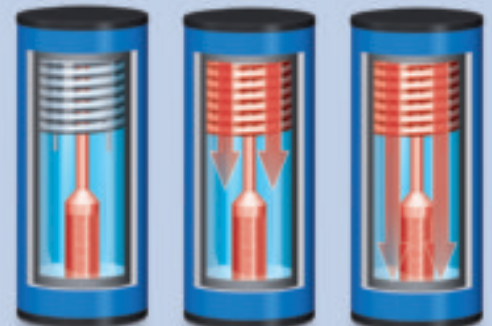
Solare Erwärmung des Speichers Logalux SL
