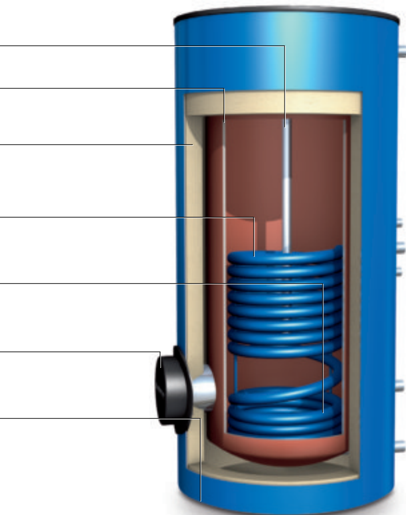
Logalux SU
