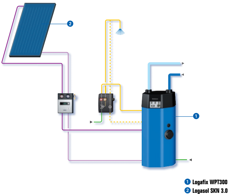
Hydraulisches Systembeispiel
