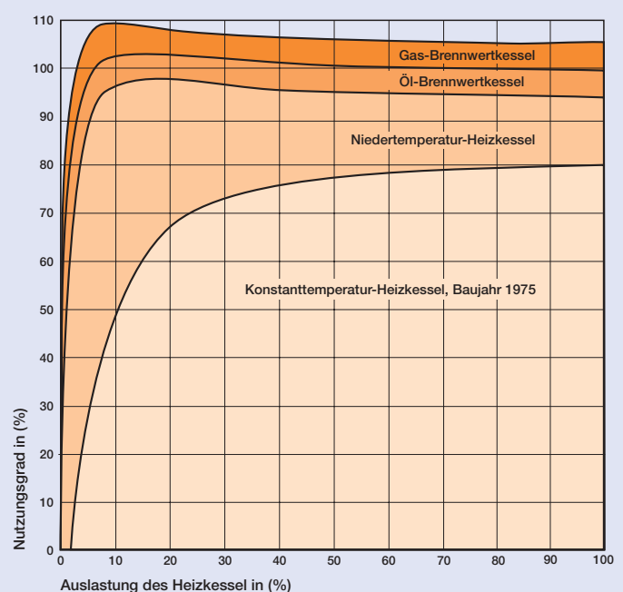
Bild 1: Teillast-Nutzungsgradverläufe von Heizkesseln
