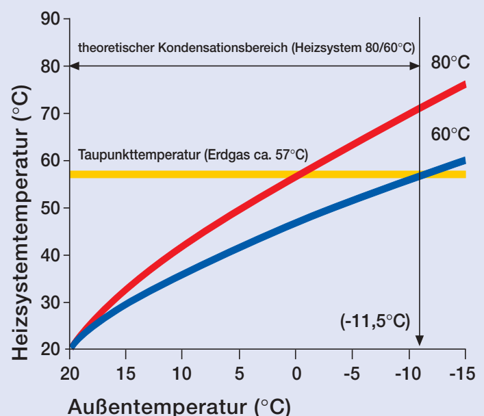
Bild 2: Gas-Brennwertnutzen bei Heizsystem 80/60^\circ\text{C}
