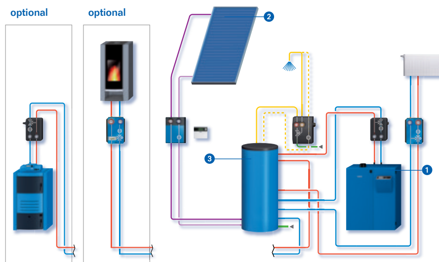
Hydraulisches Systembeispiel
