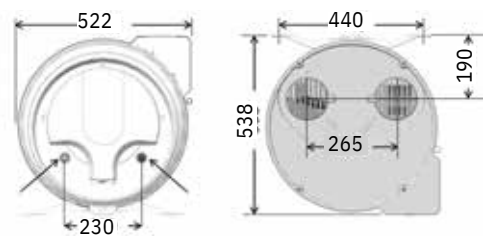
Ansicht unten
