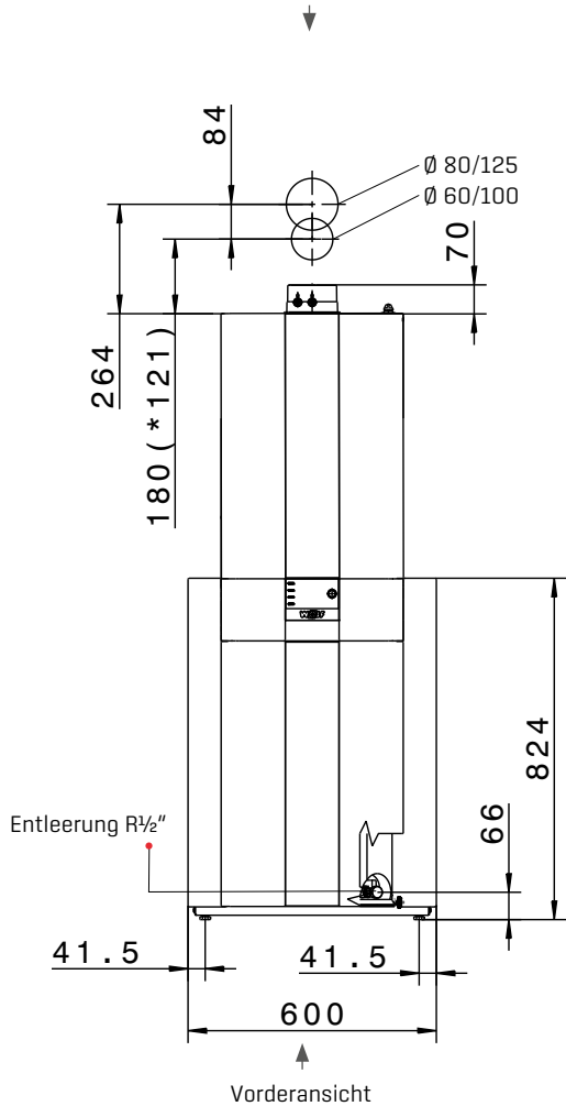
Vorderansicht
