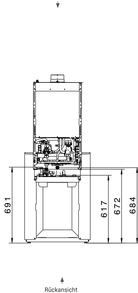
Rückansicht
