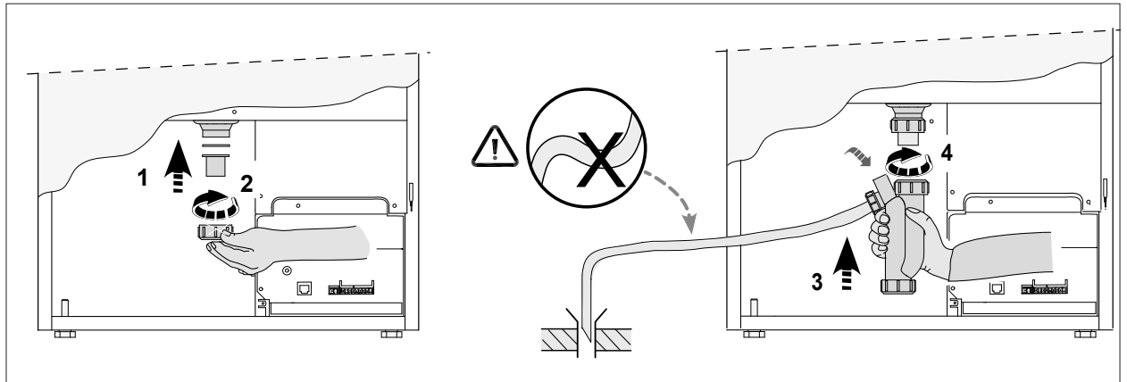
Abb. 11.22 Siphon montieren
