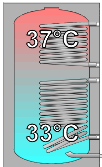
Zerstörte Temperaturschichtung
